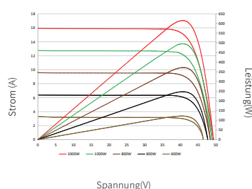
Strom-Spannungs- und Leistungs-Spannungs-Diagramme(615W)
